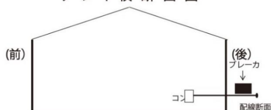
テント横断面図
